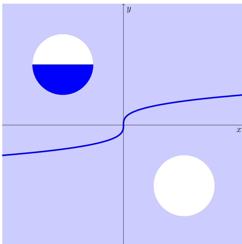
RYSUNEK 5. y = \sqrt[3]{x} na (-8, 8) oraz dwa koła
