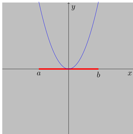
RYSUNEK 4. y = x^2 na (-2.25, 2.25)
